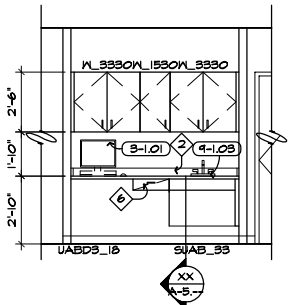
2 CHECK-IN - 122 SCALE: 1/4" = 1'-0"
