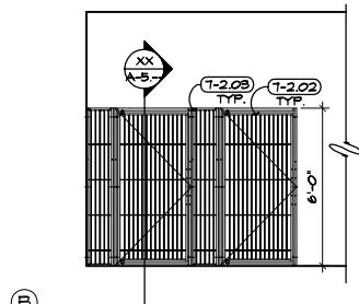
5 DOG 150 - 117 SCALE: 1/4" = 1'-0"
