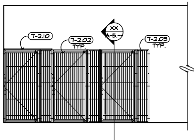
6 DOG HOLD / QUAR. - 118 SCALE: 1/4" = 1'-0"
