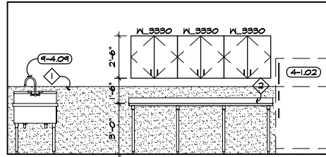
1 UTILITY - 119 SCALE: 1/4" = 1'-0"
