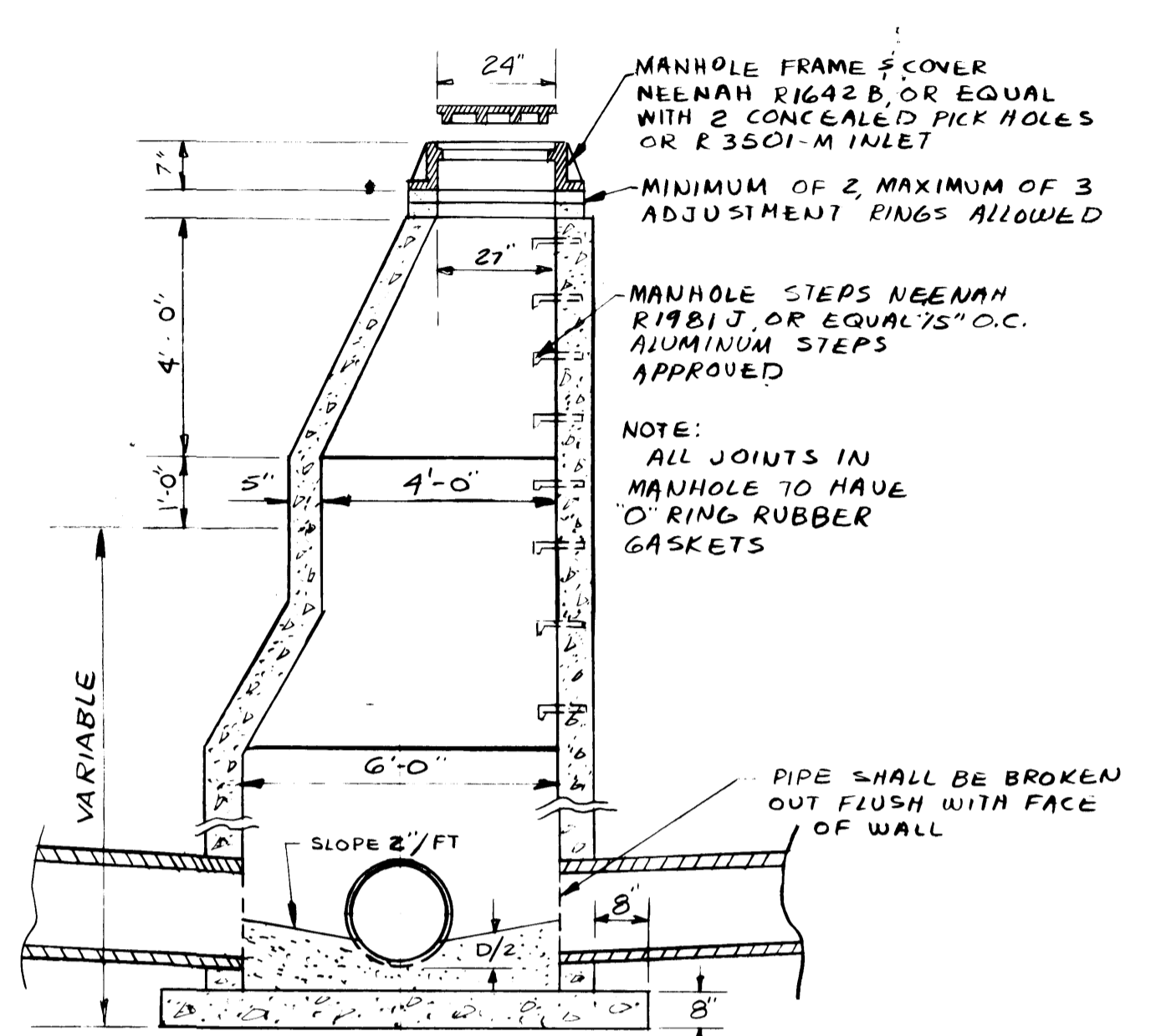
DETAIL SECTION VIEW 6 FT MANHOLE N.T.S.
